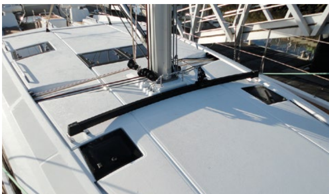
Self-tacking jib or staysail / Foc ou Trinquette sur rail auto vireur
