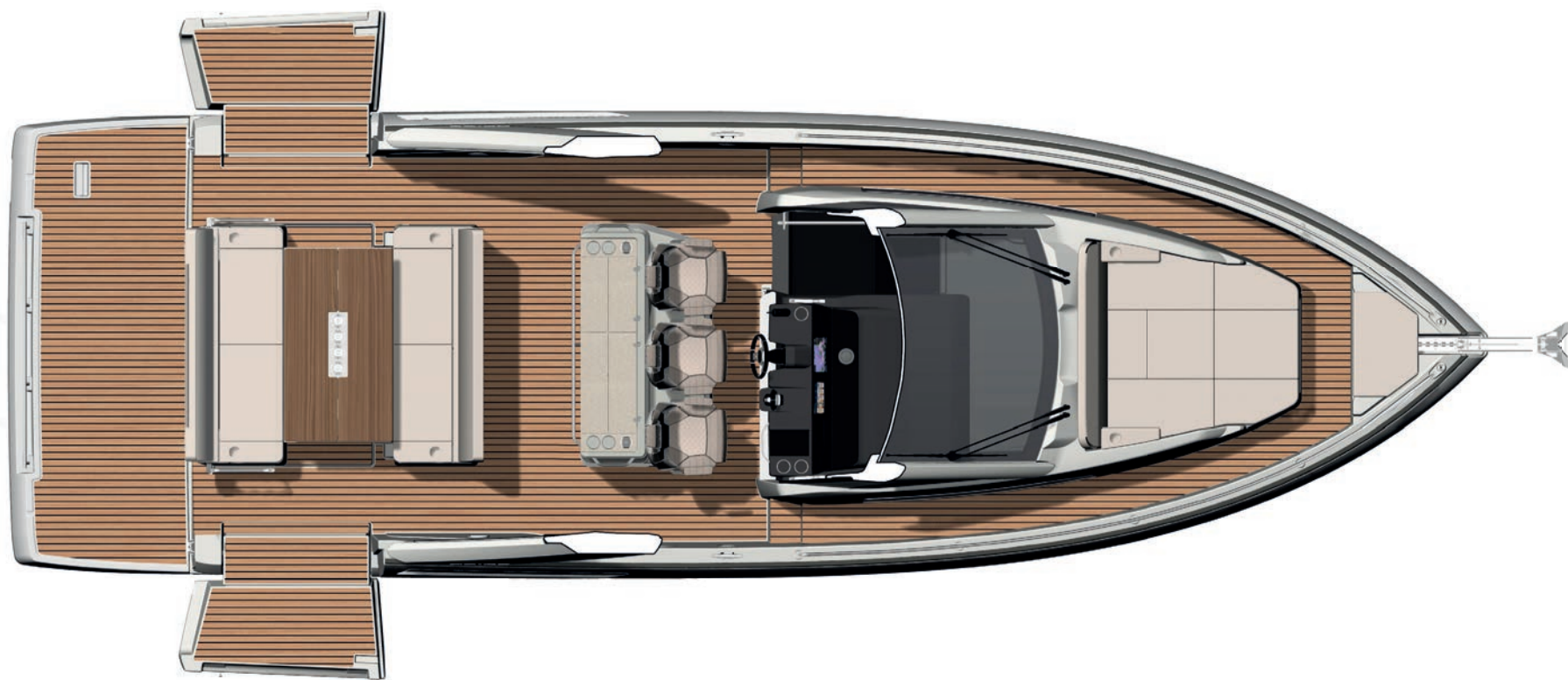
Version inbord / Inboard version : Aménagement extérieur / Exterior Layout
